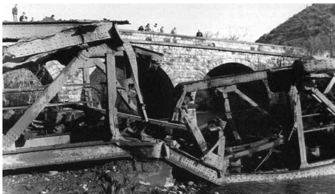
Слика 2. Срушени железнички мост Лопатница, поред каменог аутомобилског моста. 40
